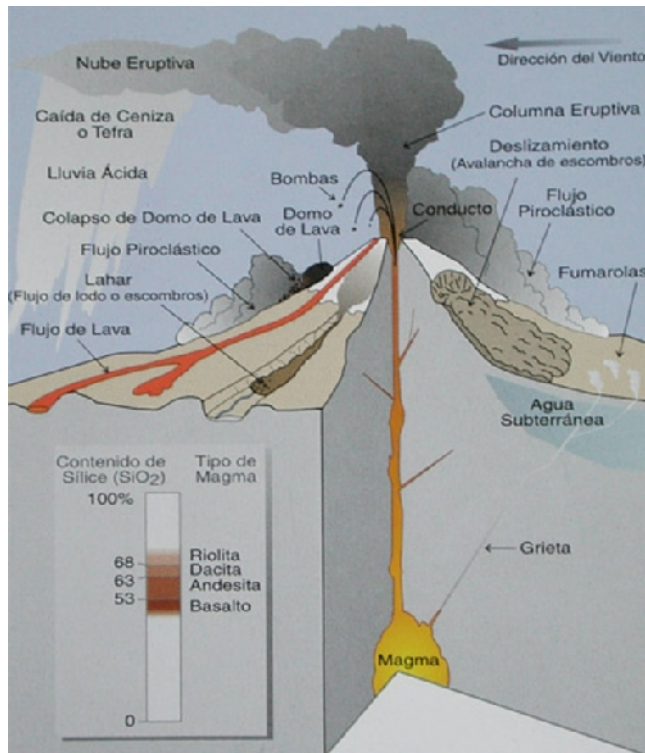
Figura 17. Partes constitutivas de un volcán.
